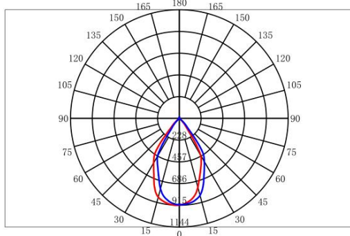
配光曲线
