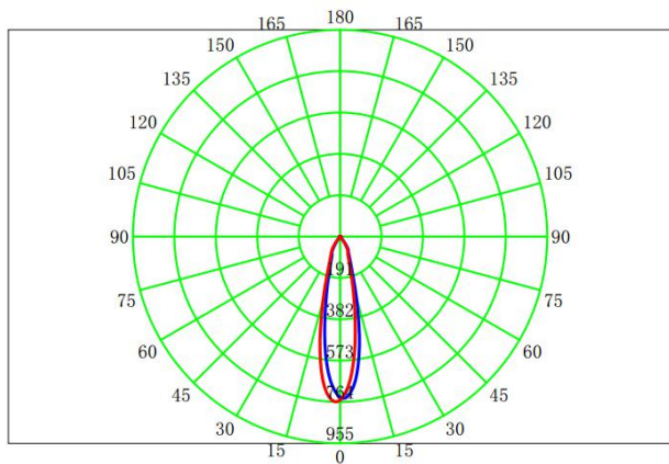
配光曲线
