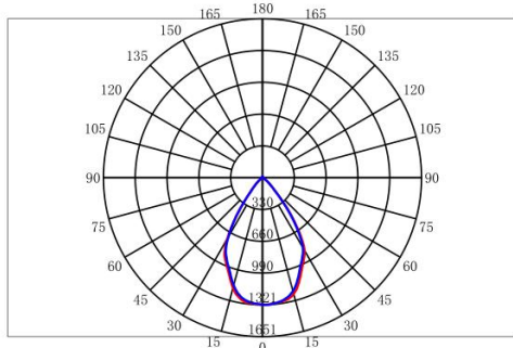
配光曲线
