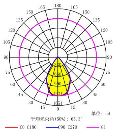
配光曲线
