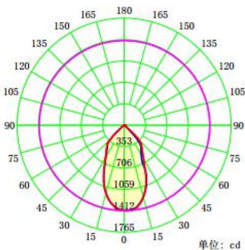
配光曲线
