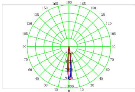
配光曲线
