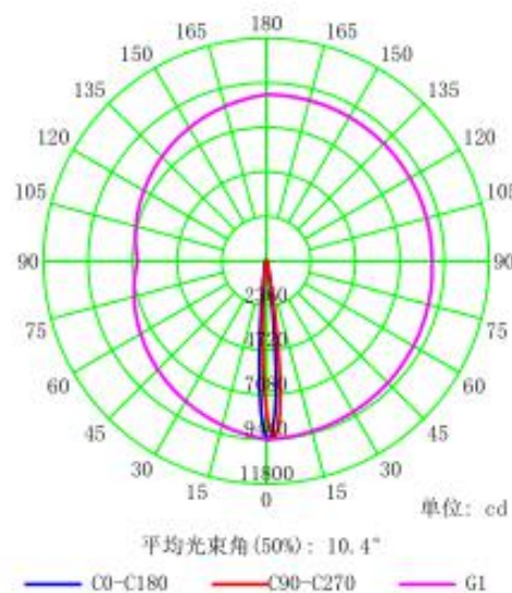
配光曲线
