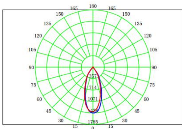
配光曲线
