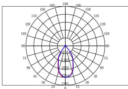
配光曲线
