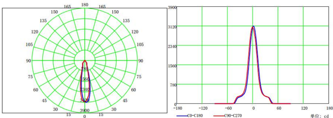
配光曲线
