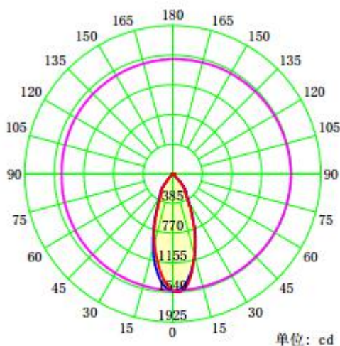
配光曲线
