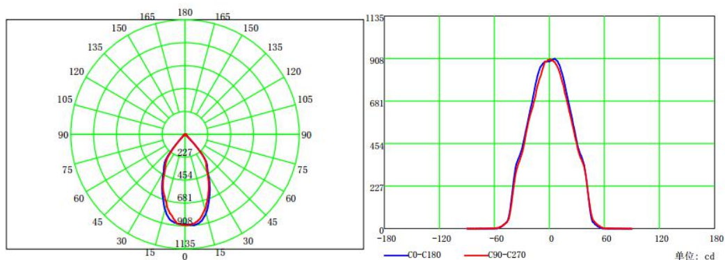
配光曲线
