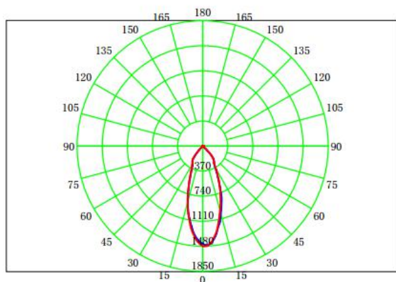
配光曲线
