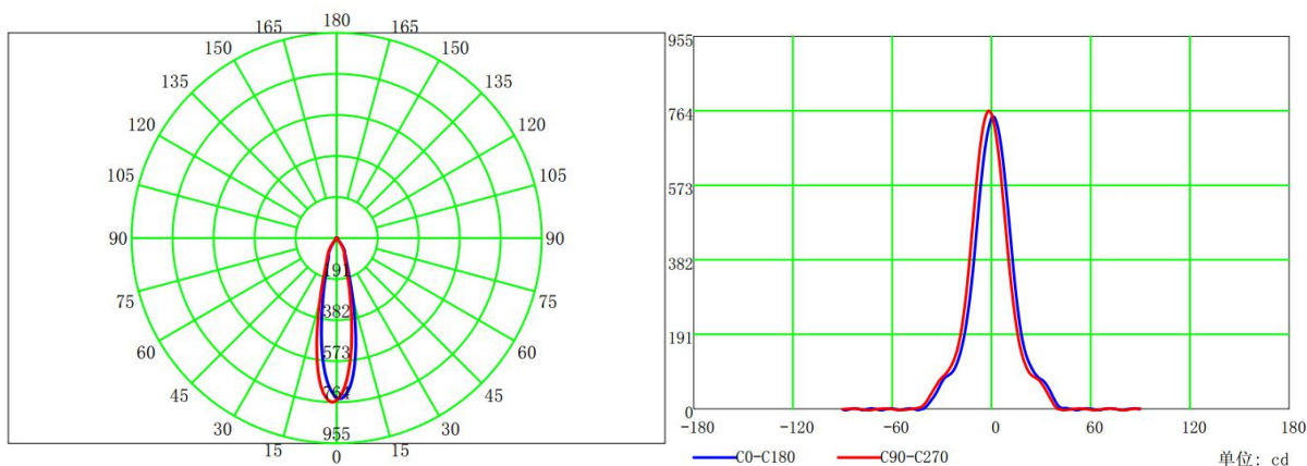
配光曲线
